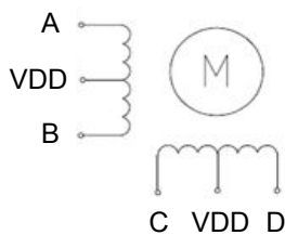
unipolaire : 6 fils
