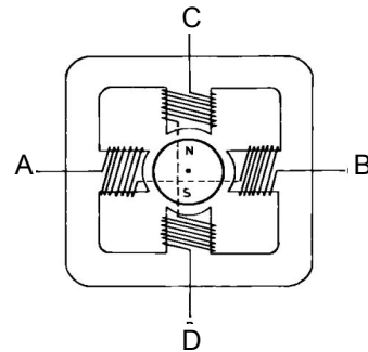
bipolaire : 4 fils
