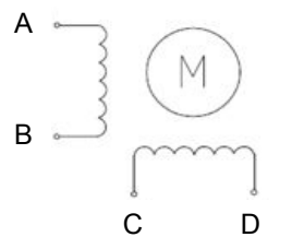
bipolaire : 4 fils
